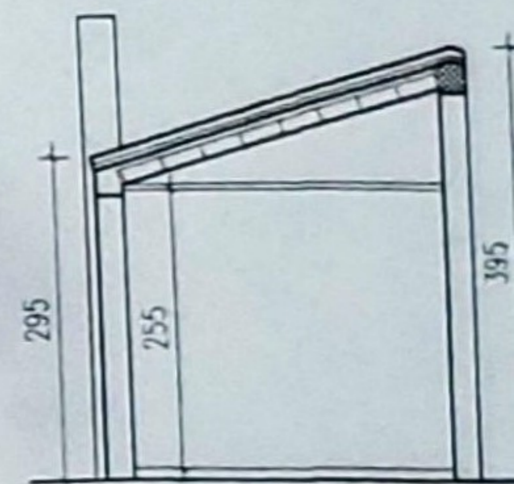
PRESJEK 3-3
