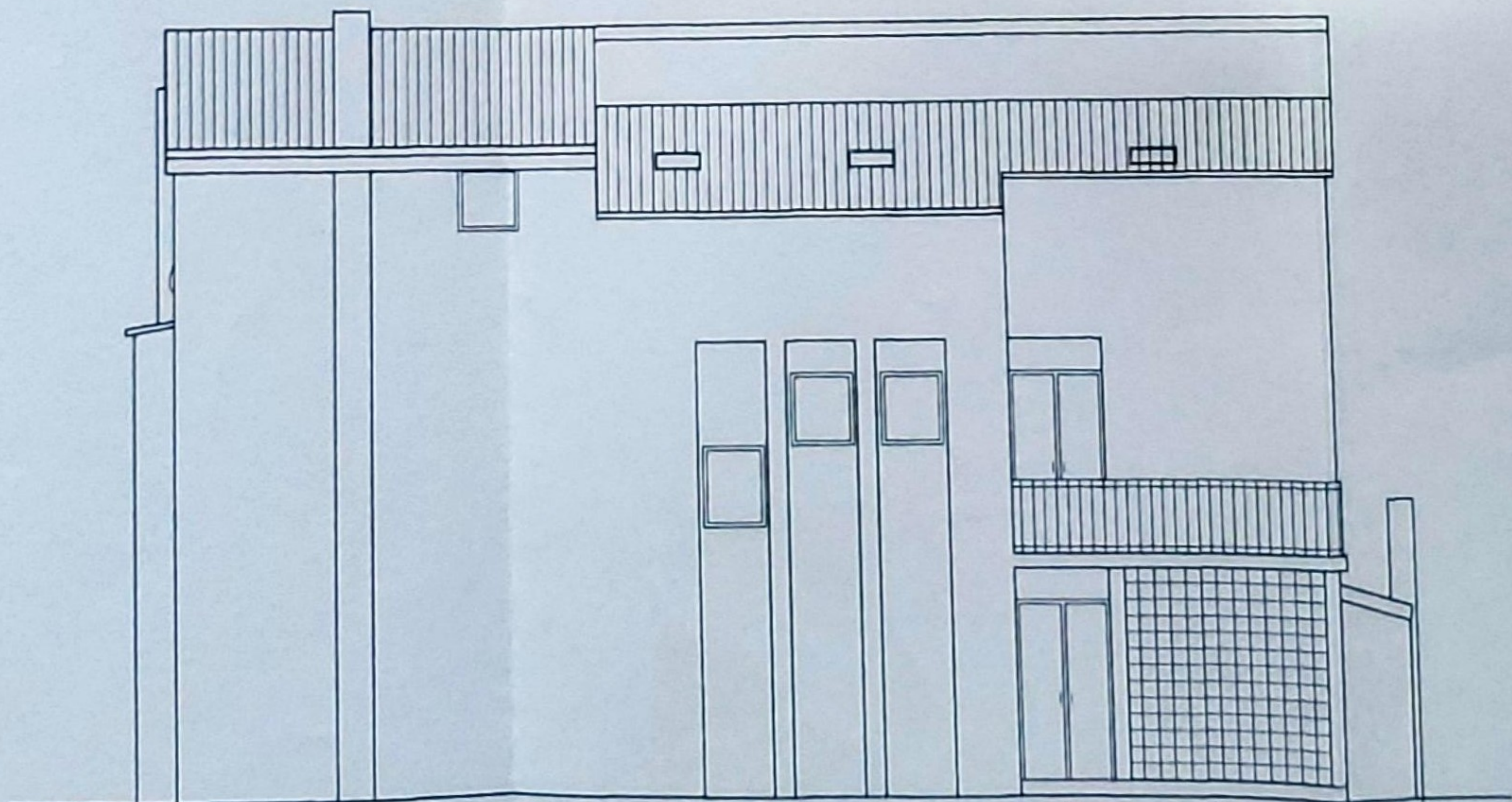
ISTOČNO PROČELJE
