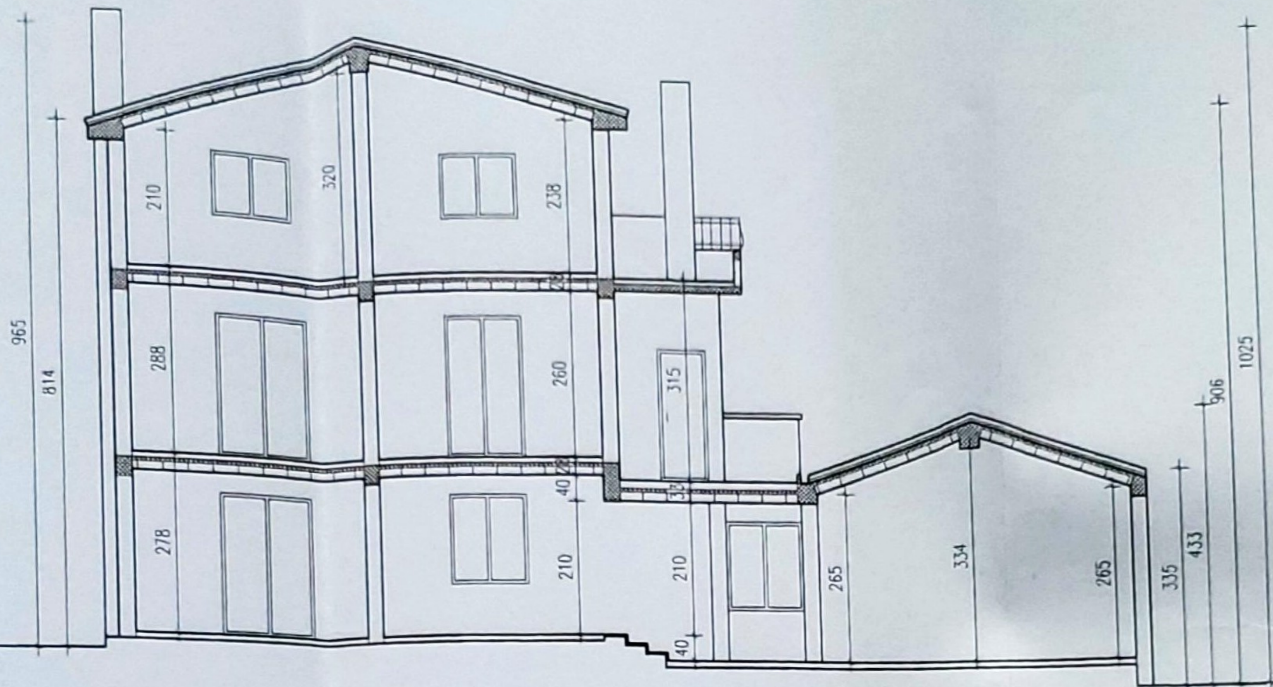
PRESJEK 1-1
