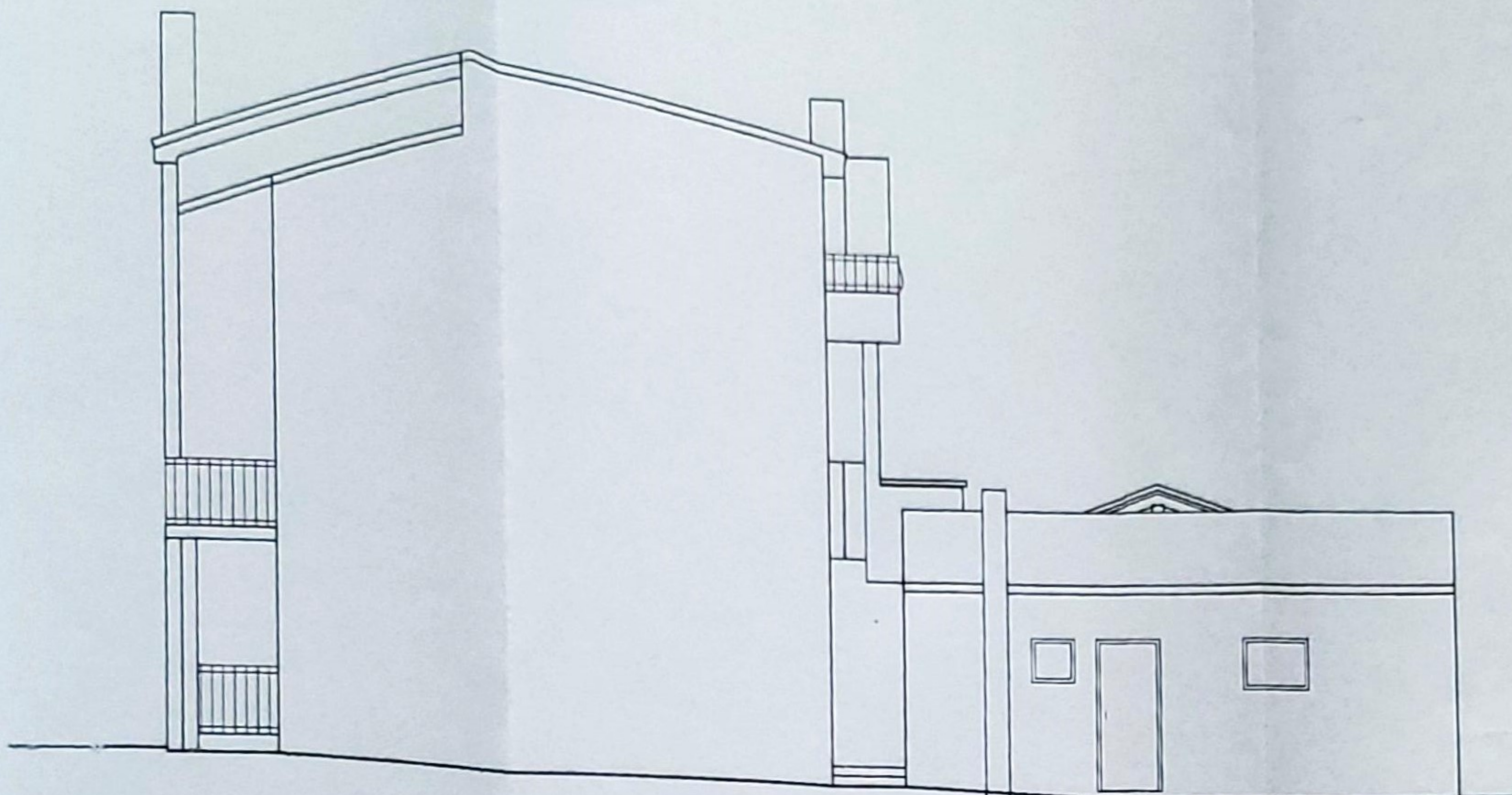
SJEVERNO PROČELJE
